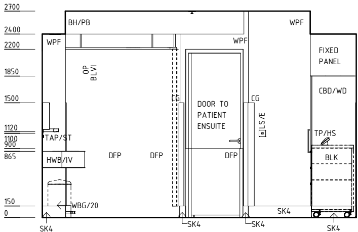
ELEVATION 3
