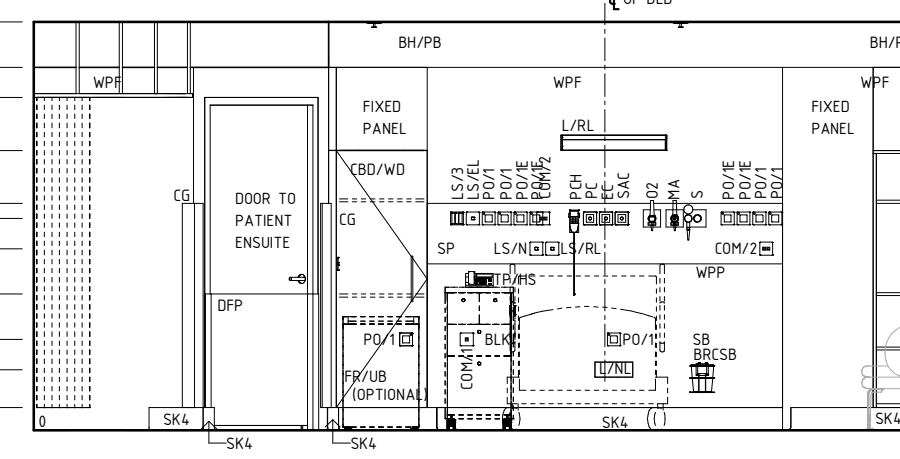
ELEVATION 4
