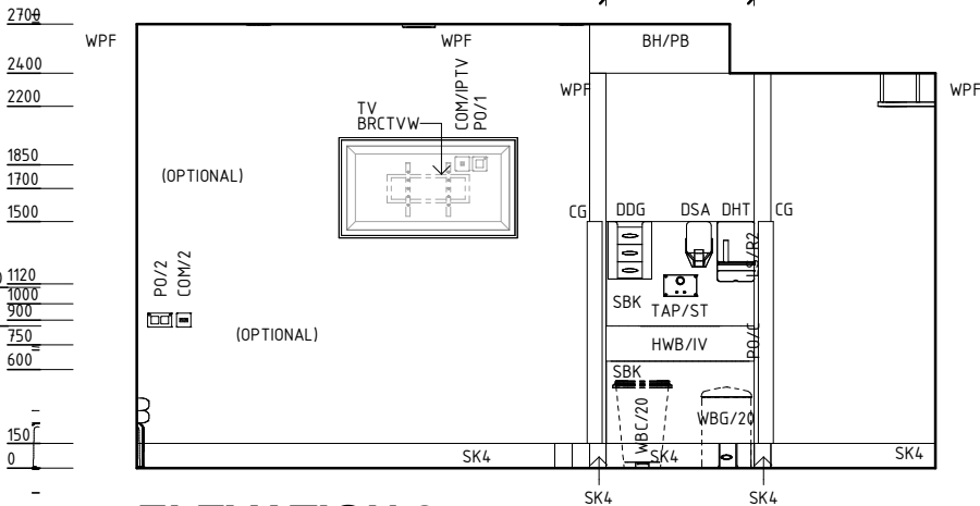
ELEVATION 2
