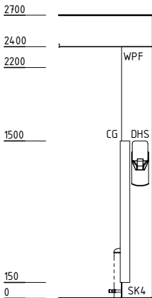
ELEVATION 5
