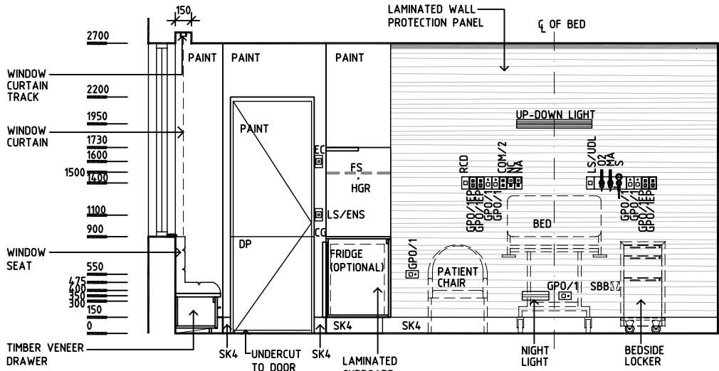
ELEVATION 2
