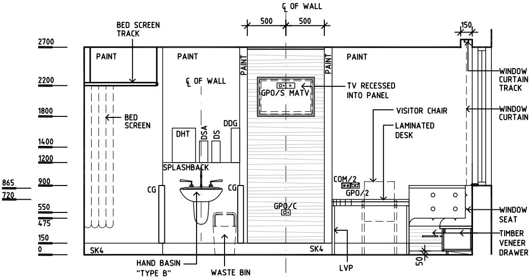
ELEVATION 4
