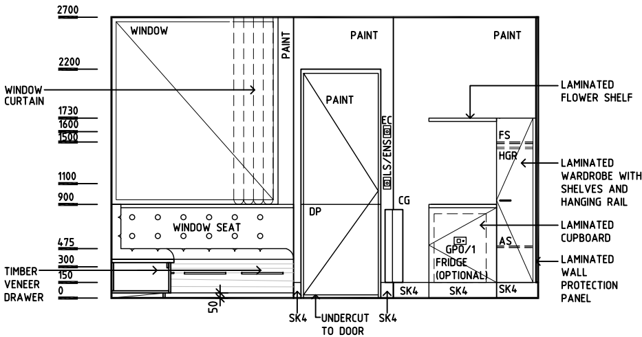
ELEVATION 1
