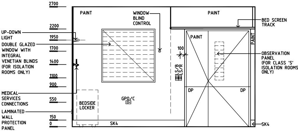
ELEVATION 3
