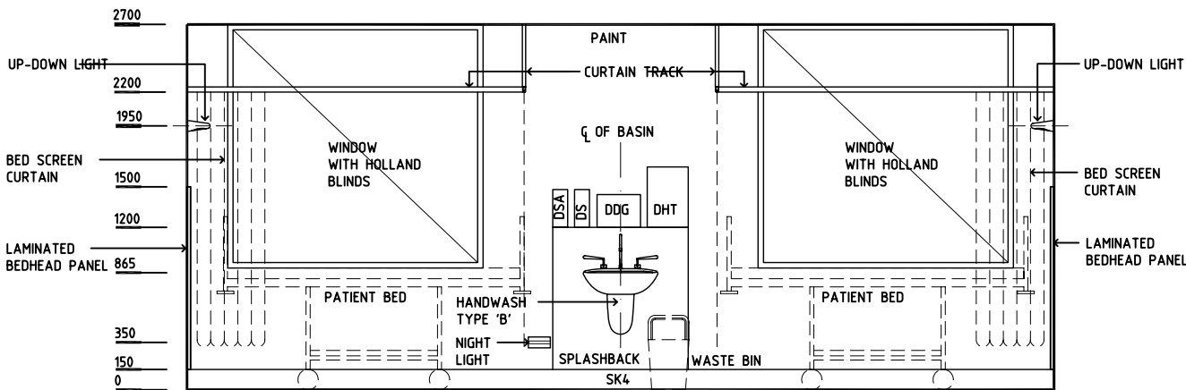
ELEVATION 4
