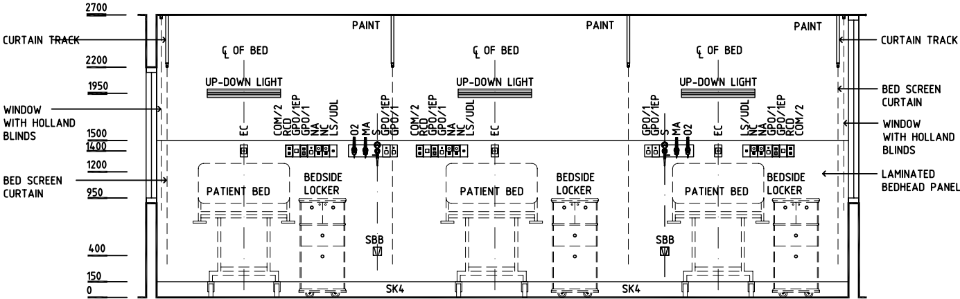
ELEVATION 3
