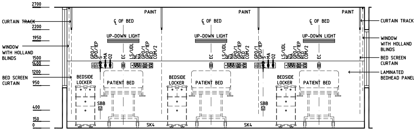
ELEVATION 1
