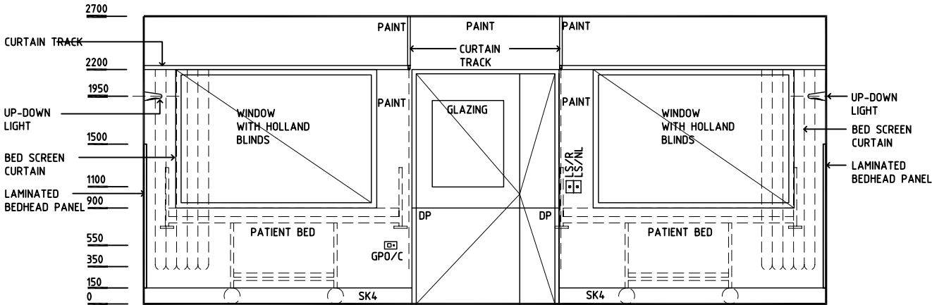
ELEVATION 2
