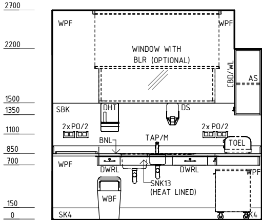
ELEVATION 1
