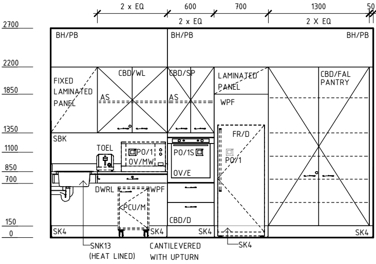
ELEVATION 2
