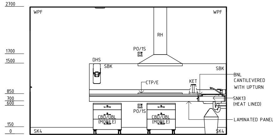
ELEVATION 4
