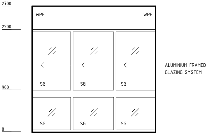
ELEVATION 2
