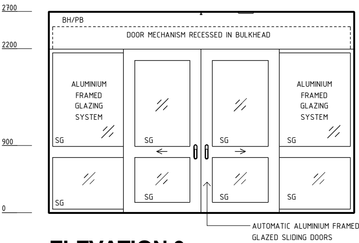
ELEVATION 3
