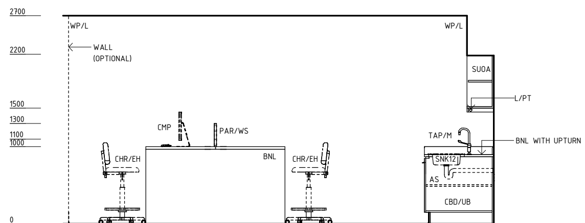
ELEVATION 3
