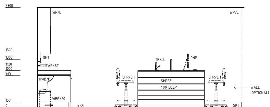
ELEVATION 6
