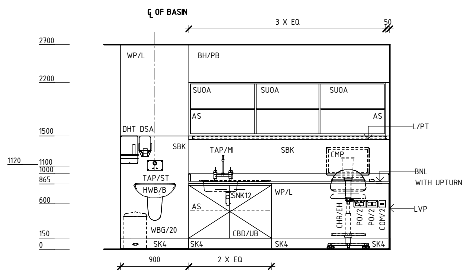
ELEVATION 4
