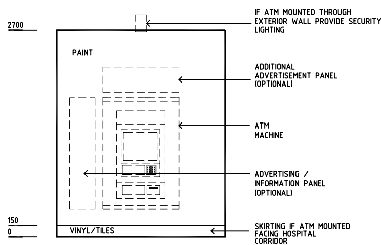
ELEVATION 3
