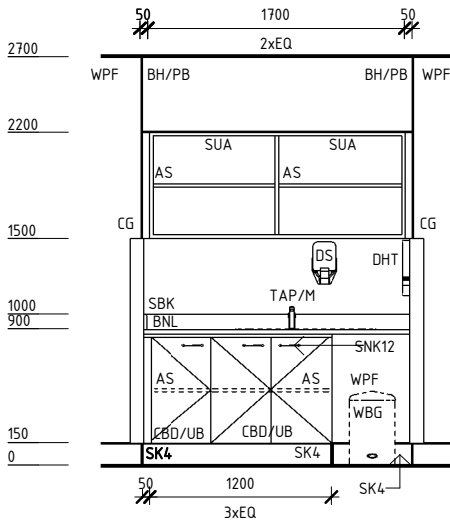
ELEVATION 2
