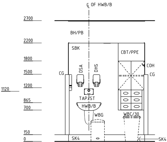
ELEVATION 1
