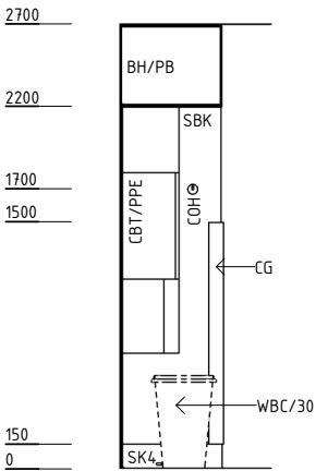
ELEVATION 2
