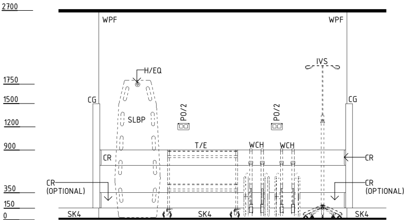
ELEVATION 1
