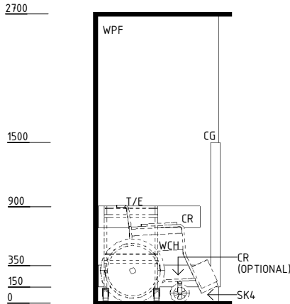
ELEVATION 2
