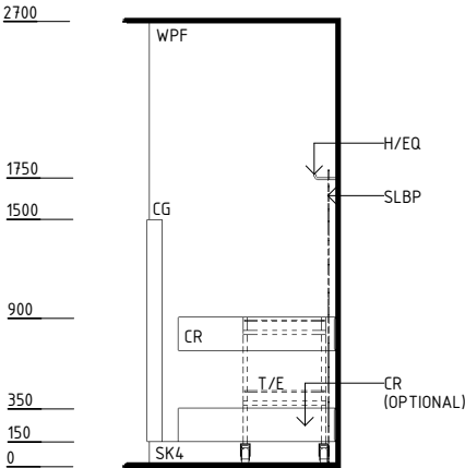
ELEVATION 3
