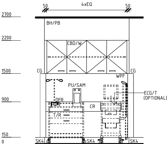
ELEVATION 2
