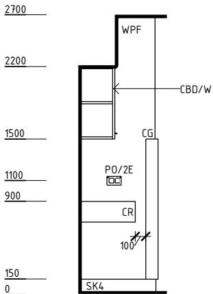
ELEVATION 3
