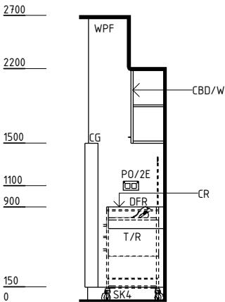
ELEVATION 1
