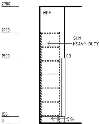
ELEVATION 2
