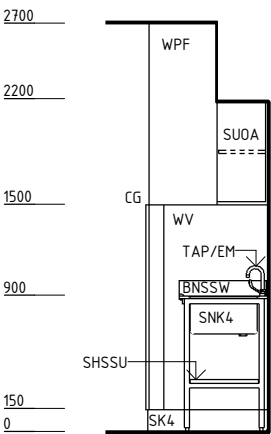
ELEVATION 1
