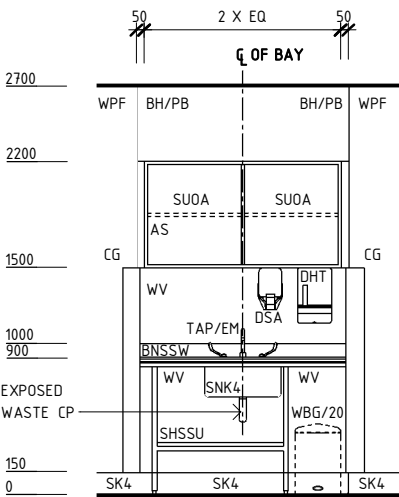
ELEVATION 2
