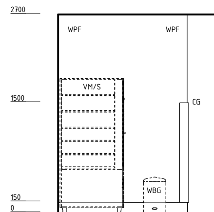
ELEVATION 3
