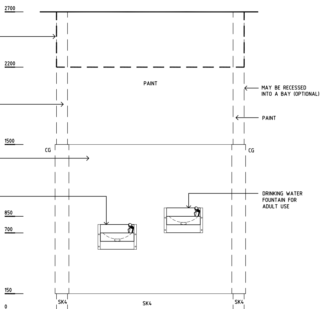
ELEVATION 2
