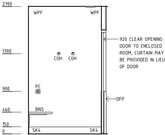
ELEVATION 2
