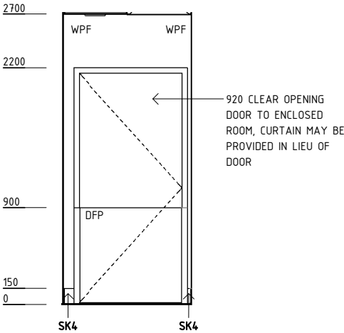
ELEVATION 3
