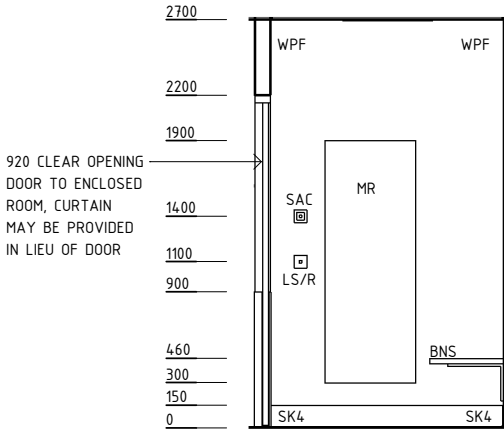
ELEVATION 4
