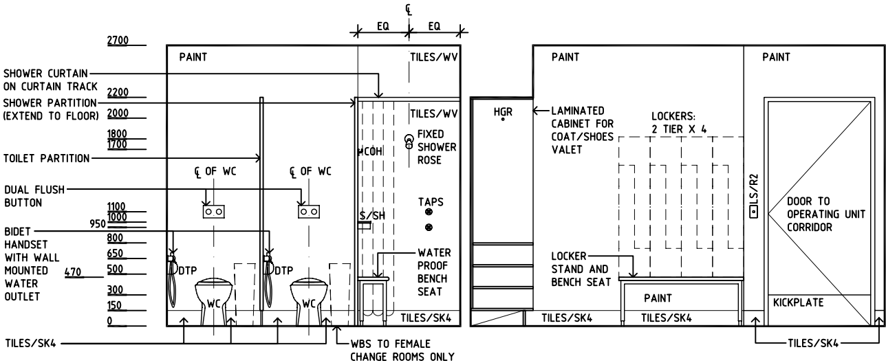
ELEVATION 4
