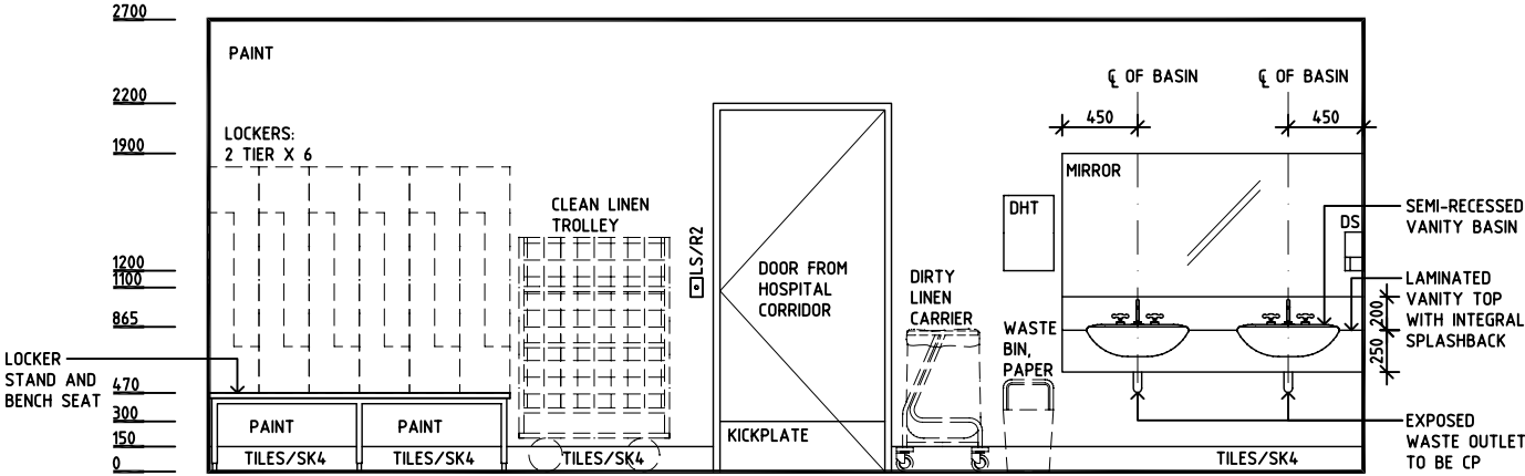
ELEVATION 2
