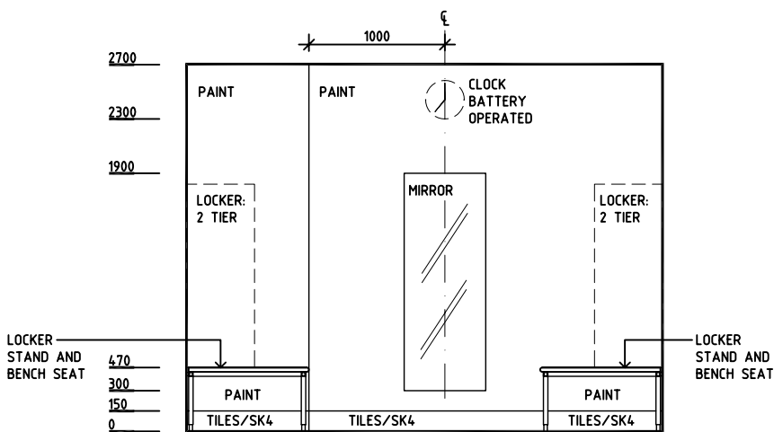
ELEVATION 1
