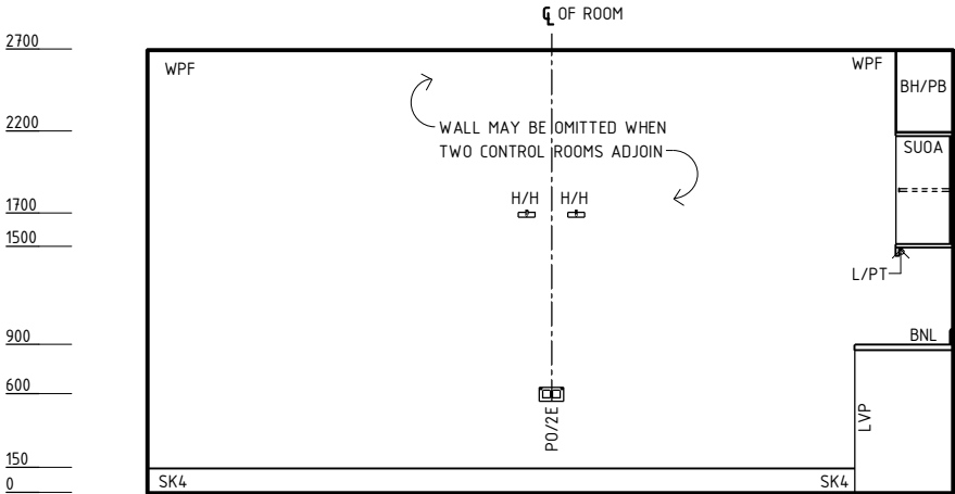
ELEVATION 4
