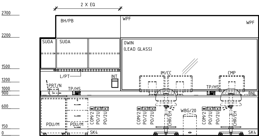
ELEVATION 2
