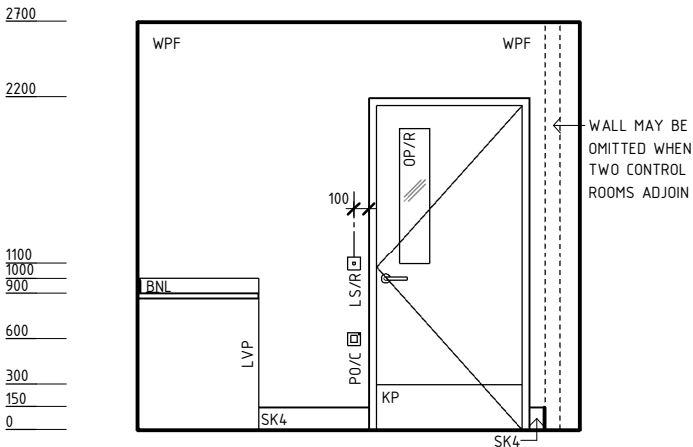
ELEVATION 3
