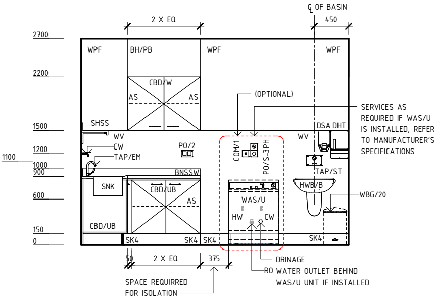
ELEVATION 2
