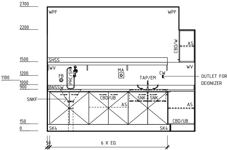
ELEVATION 1
