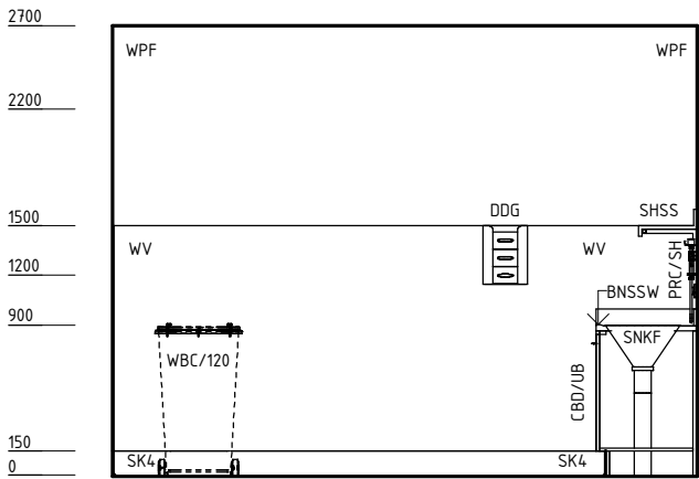
ELEVATION 4
