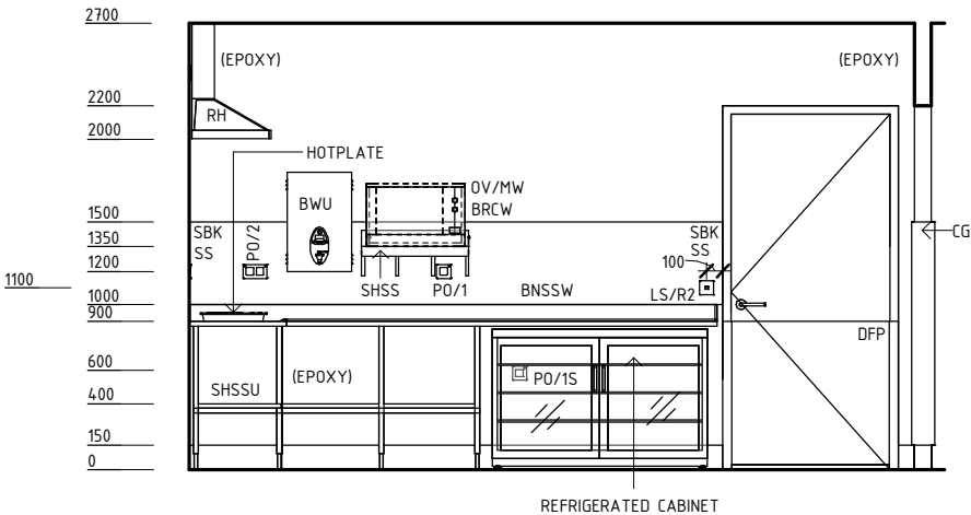
ELEVATION 1
