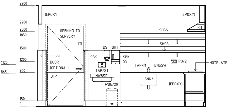
ELEVATION 3
