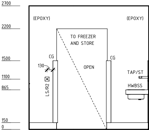
ELEVATION 2
