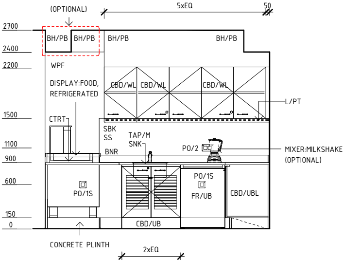
ELEVATION 4
