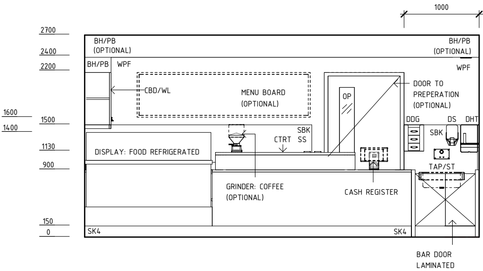
ELEVATION 5
