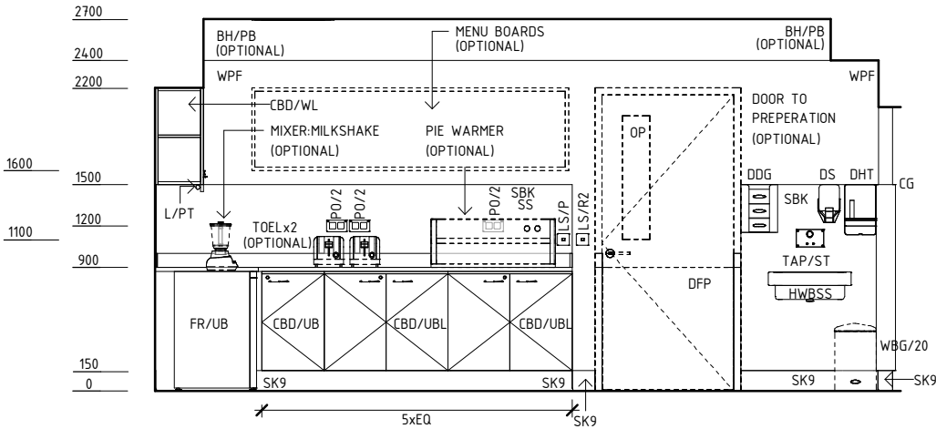
ELEVATION 1
