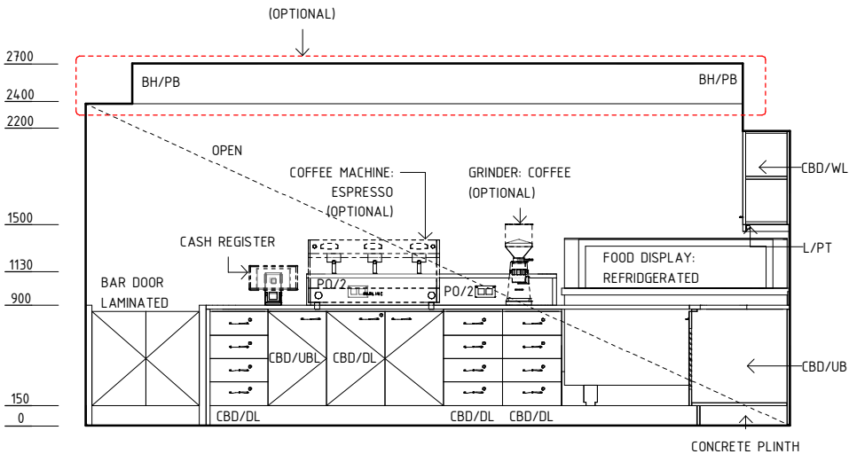
ELEVATION 3
