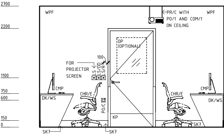
ELEVATION 3
