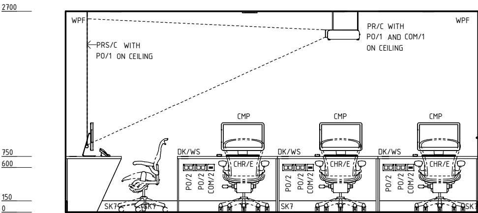
ELEVATION 2
