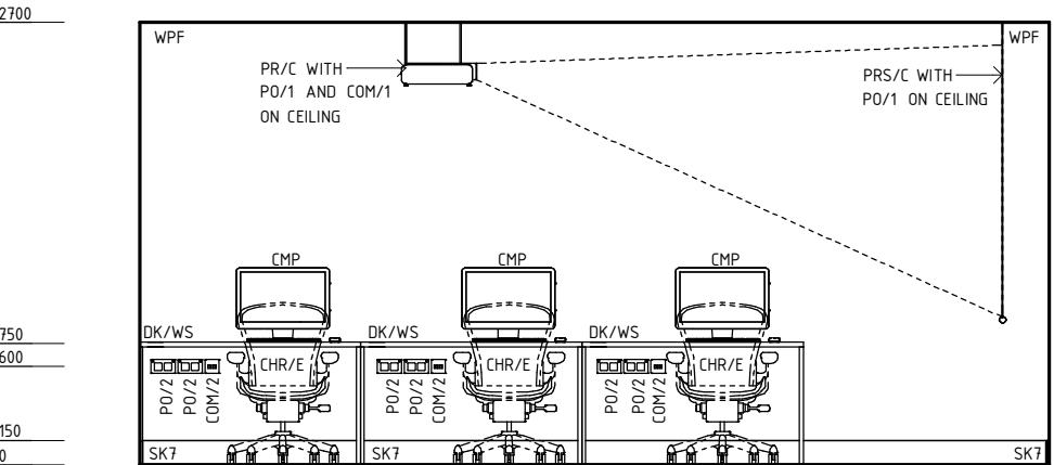
ELEVATION 4
