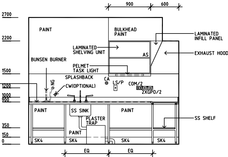
ELEVATION 4
