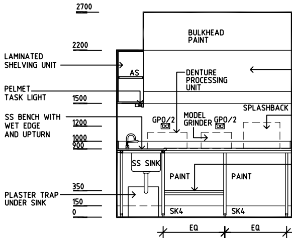
ELEVATION 1
