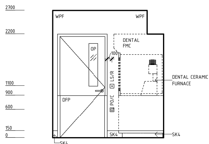
ELEVATION 3
