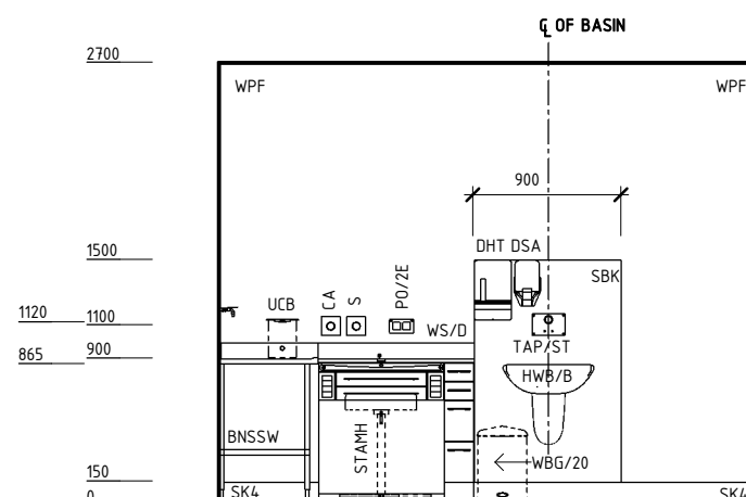
ELEVATION 2
