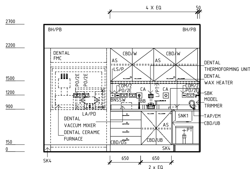
ELEVATION 4
