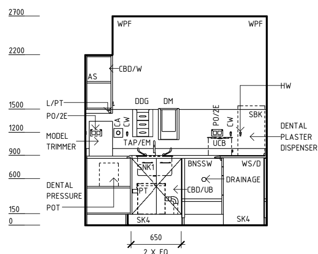
ELEVATION 1
