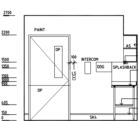
ELEVATION 3
