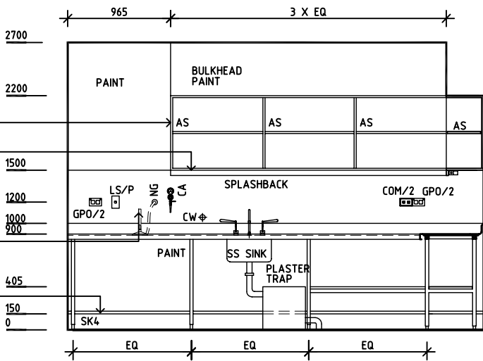
ELEVATION 4
