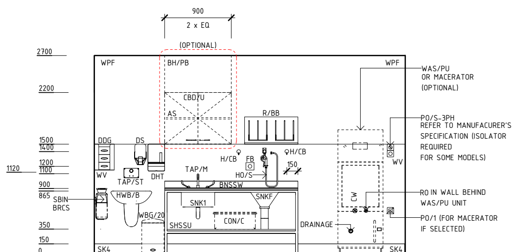
ELEVATION 4
