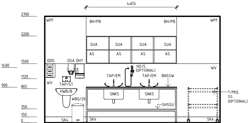
ELEVATION 4
