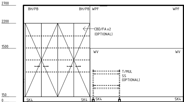
ELEVATION 2
