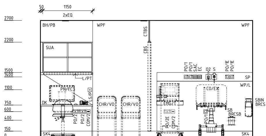
ELEVATION 4
