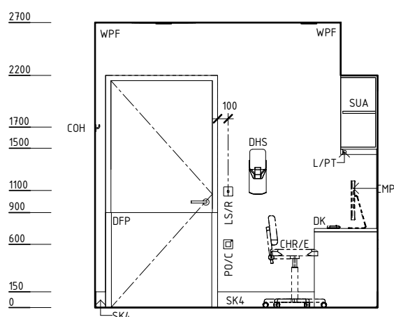
ELEVATION 3
