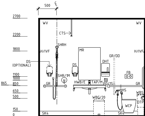
ELEVATION 2
