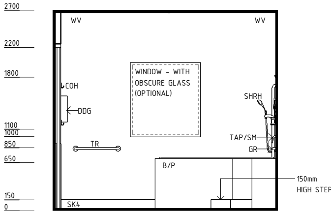
ELEVATION 4
