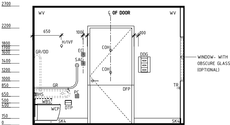
ELEVATION 3
