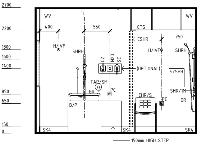
ELEVATION 1
