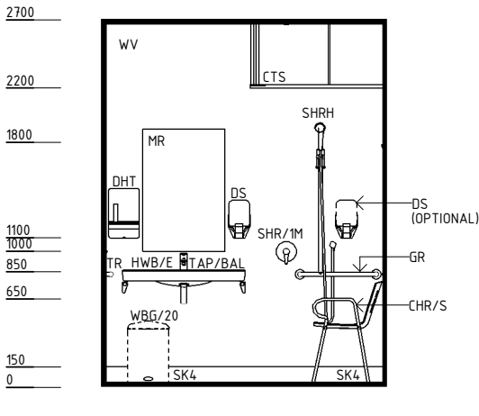
ELEVATION 4
