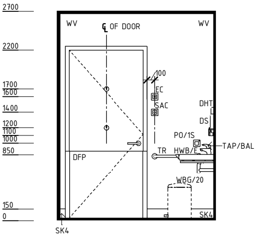
ELEVATION 3
