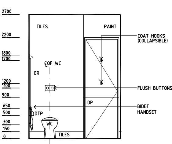
ELEVATION 4
