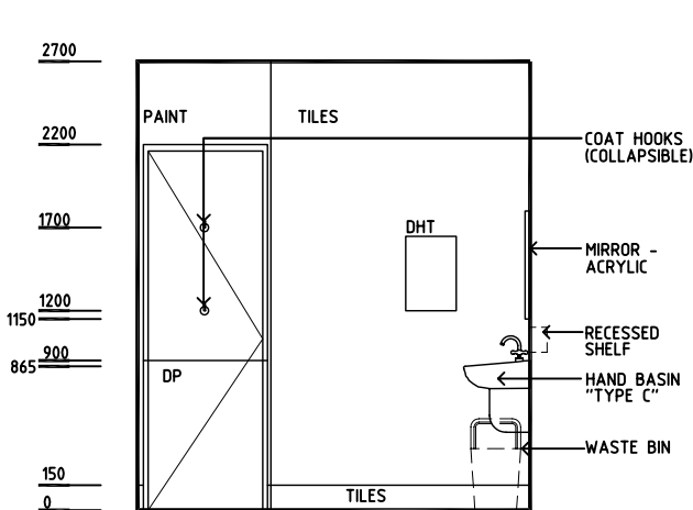
ELEVATION 1
