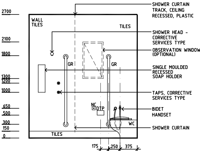
ELEVATION 3
