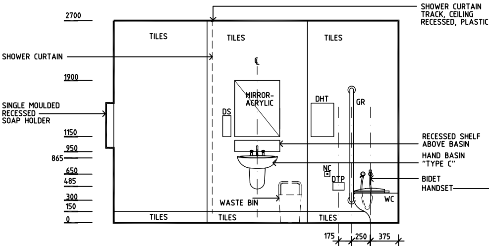
ELEVATION 1
