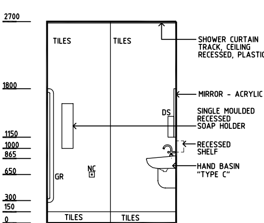
ELEVATION 4
