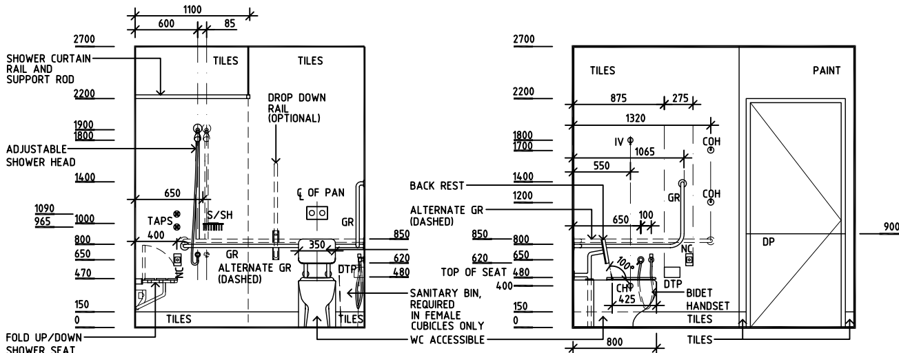
ELEVATION 3
