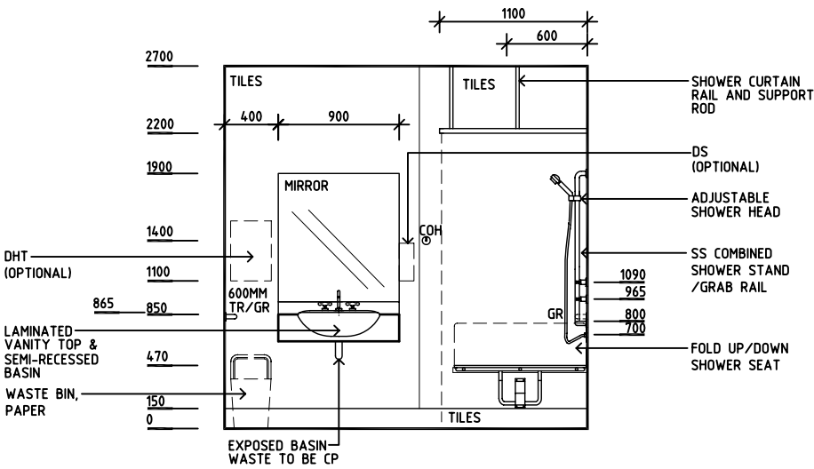
ELEVATION 2
