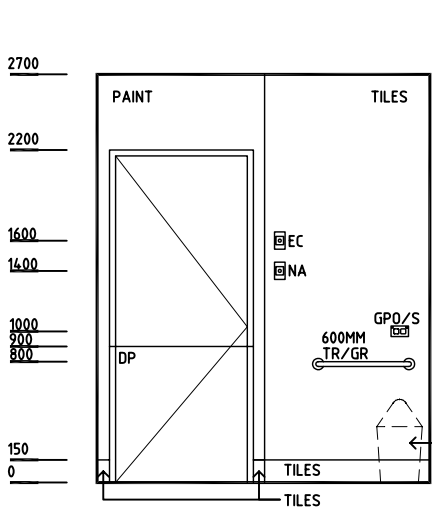
ELEVATION 1
