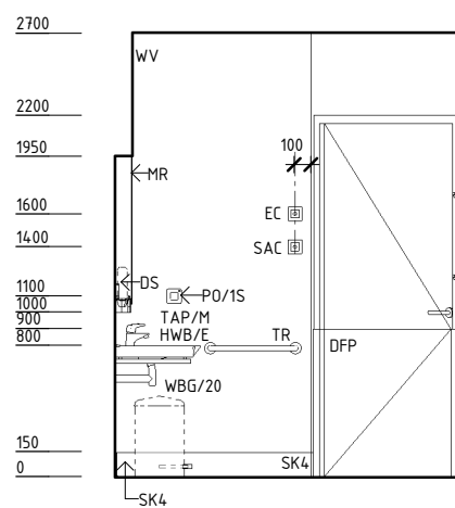
ELEVATION 1
