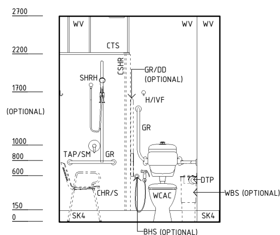
ELEVATION 3
