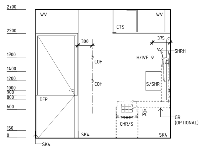
ELEVATION 2
