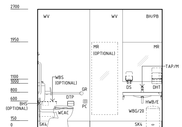
ELEVATION 4
