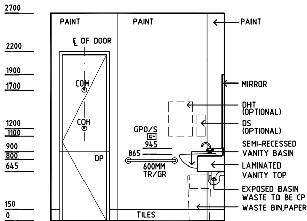
ELEVATION 4
