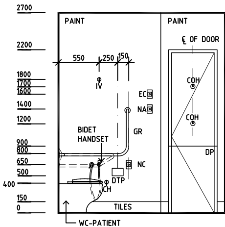
ELEVATION 3
