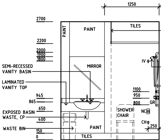
ELEVATION 1
