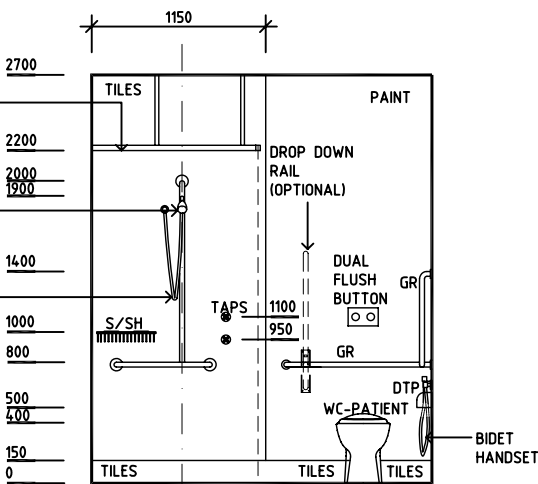
ELEVATION 2
