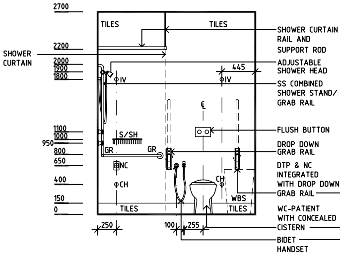
ELEVATION 3
