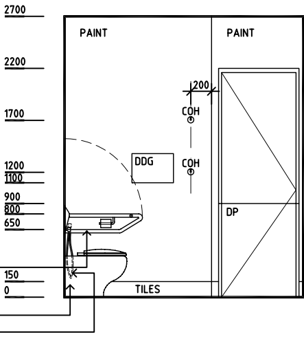
ELEVATION 4
