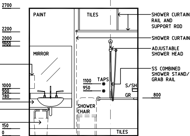
ELEVATION 2
