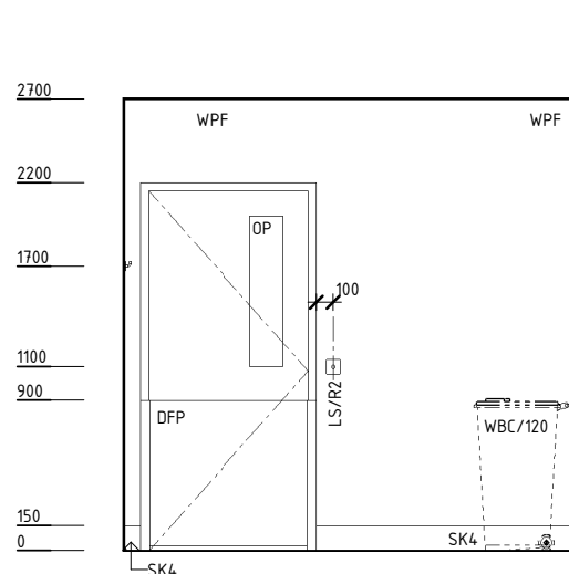
ELEVATION 1
