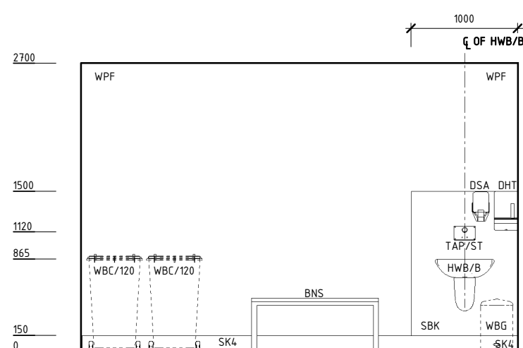
ELEVATION 2
