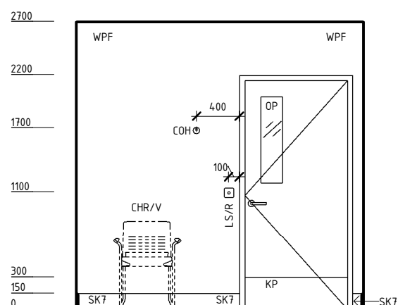
ELEVATION 3
