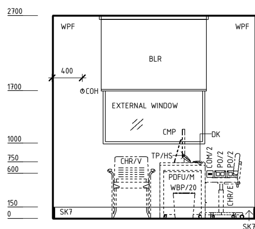
ELEVATION 1
