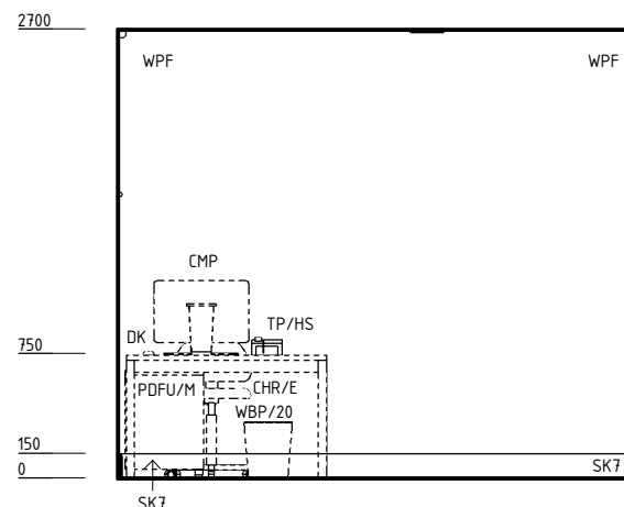
ELEVATION 2
