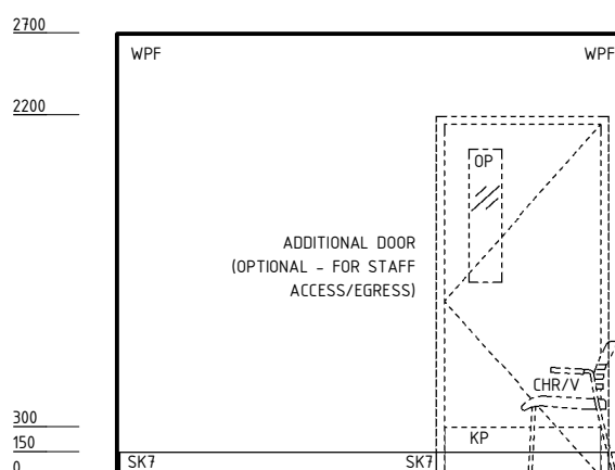
ELEVATION 4
