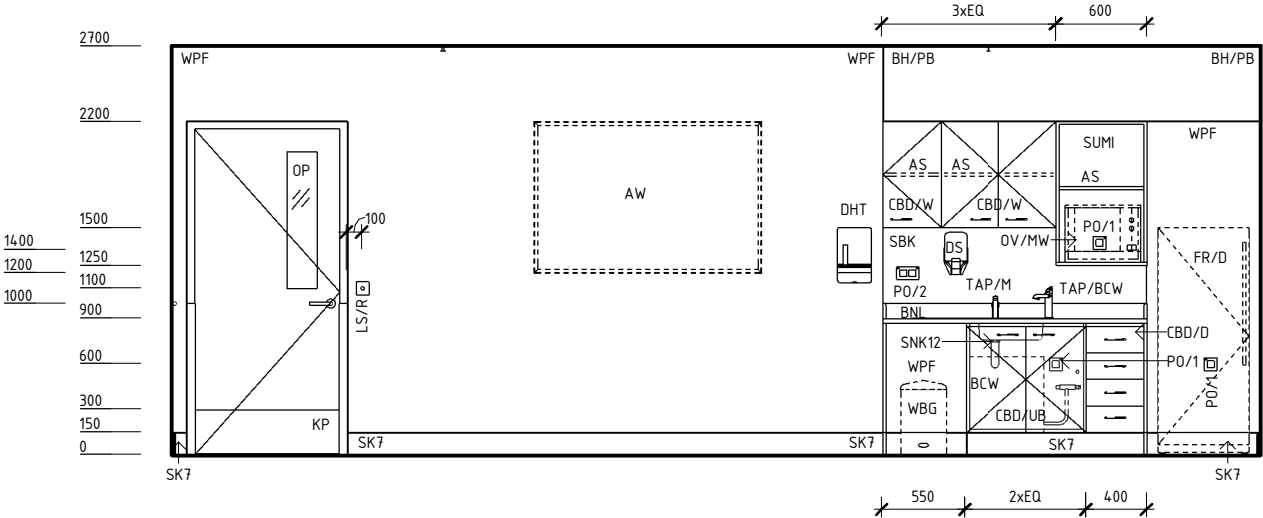
ELEVATION 3
