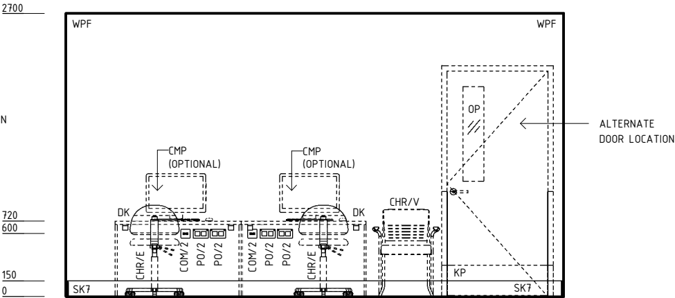
ELEVATION 2
