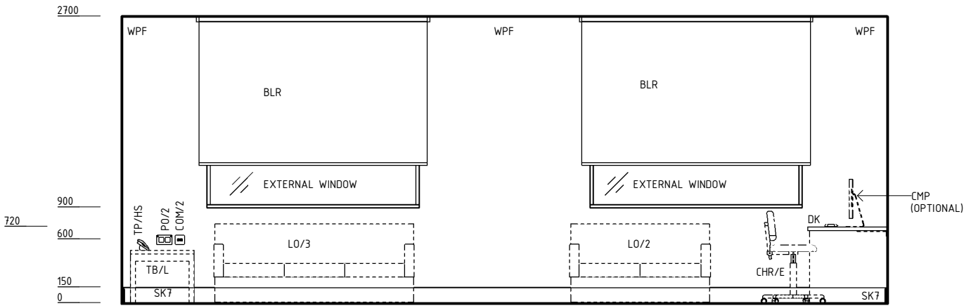
ELEVATION 1
