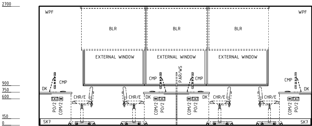
ELEVATION 1
