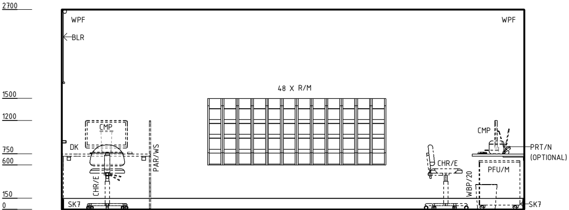
ELEVATION 2
