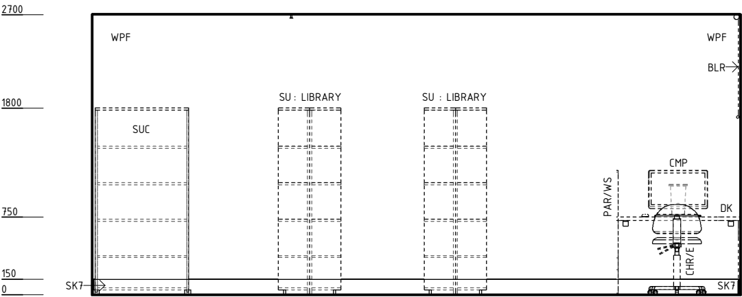
ELEVATION 4
