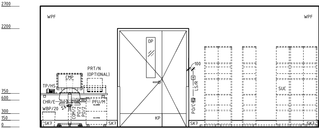
ELEVATION 3
