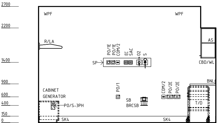
ELEVATION 1
