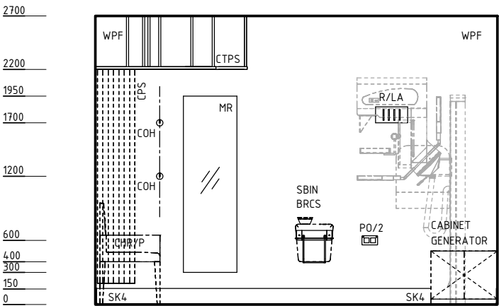
ELEVATION 4
