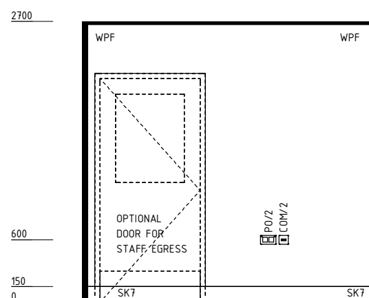
ELEVATION 4
