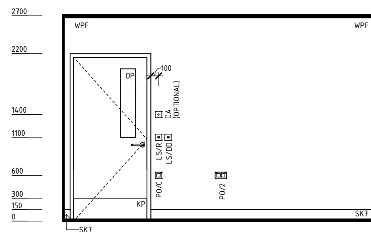
ELEVATION 3
