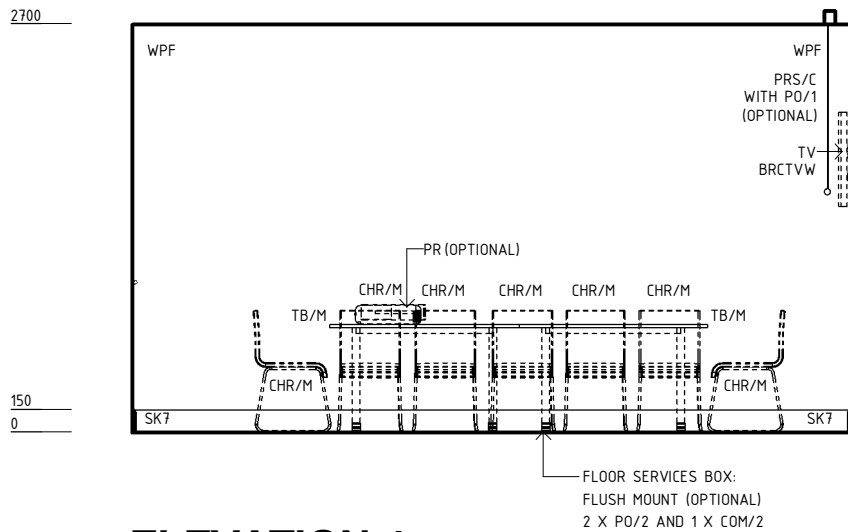
ELEVATION 4
