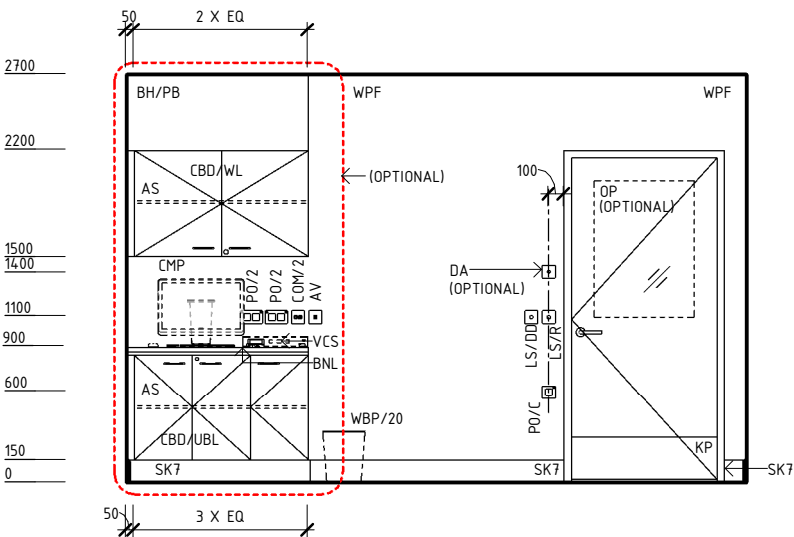
ELEVATION 3
