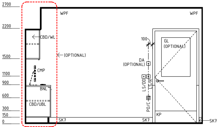
ELEVATION 3
