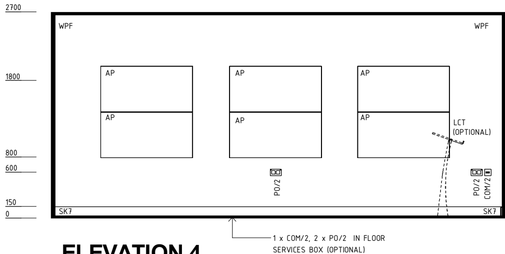
ELEVATION 4
