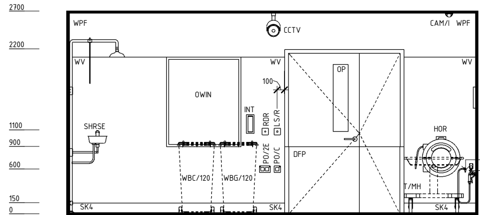
ELEVATION 3
