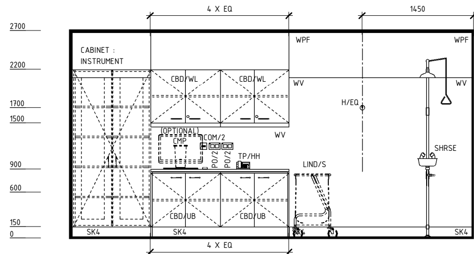
ELEVATION 2
