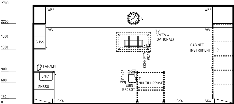
ELEVATION 1
