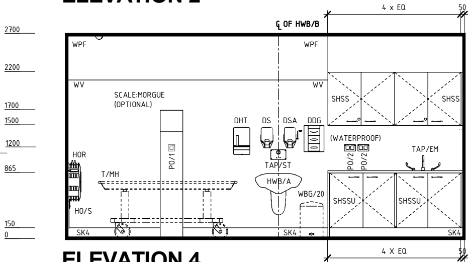
ELEVATION 4
