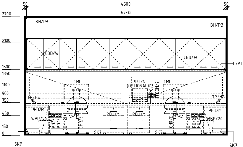
ELEVATION 2
