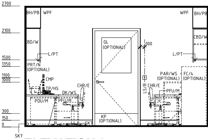
ELEVATION 3
