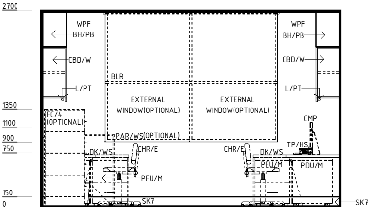
ELEVATION 1
