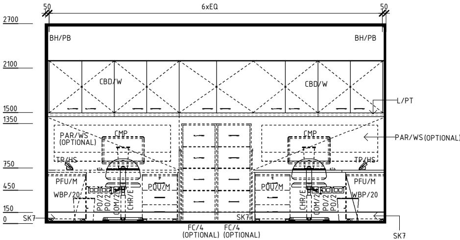
ELEVATION 4
