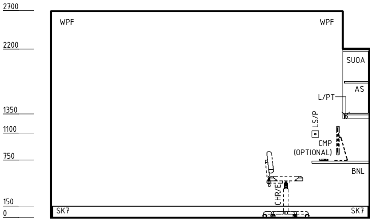
ELEVATION 4
