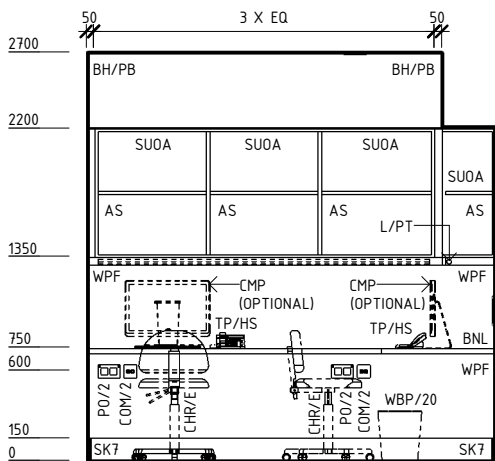
ELEVATION 1
