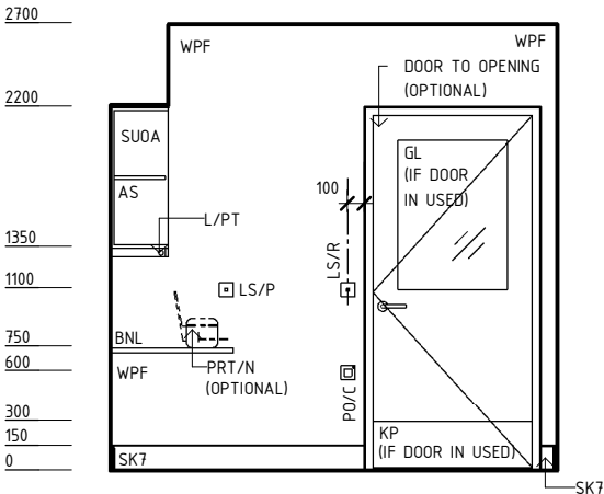
ELEVATION 3
