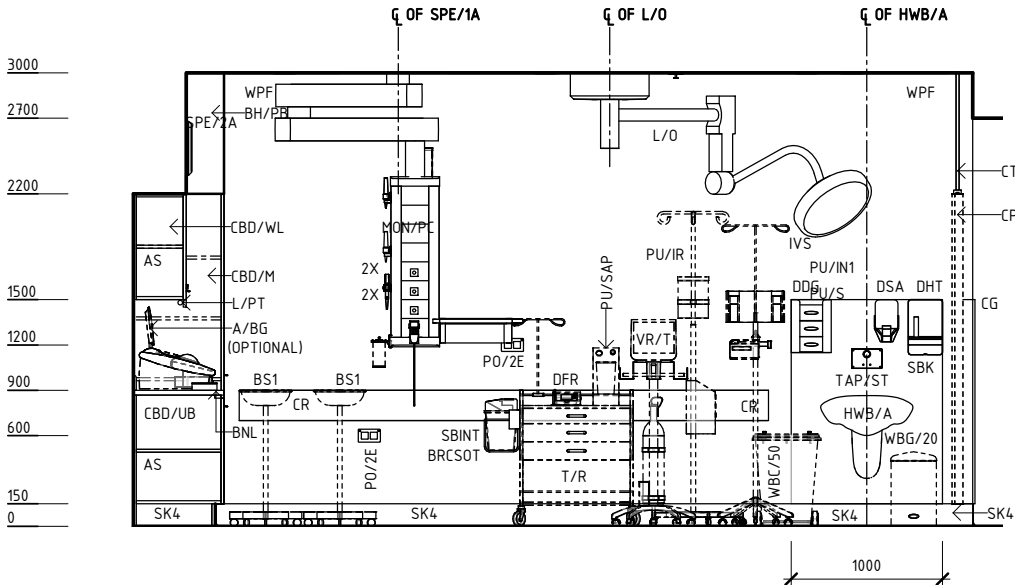
ELEVATION 1
