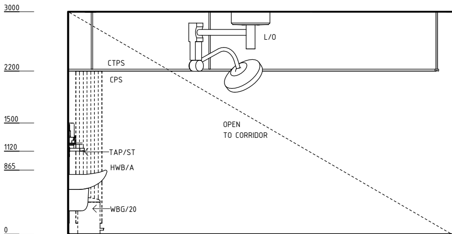
ELEVATION 2
