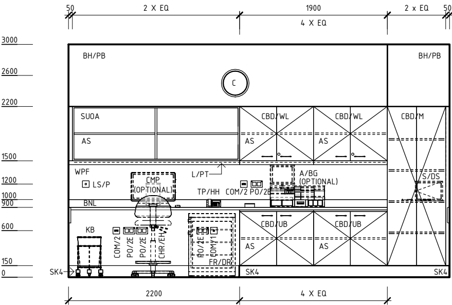
ELEVATION 4
