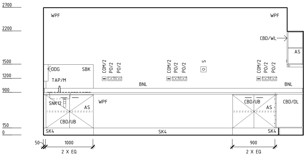
ELEVATION 01
