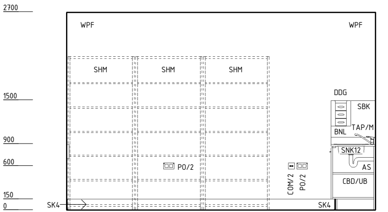
ELEVATION 04
