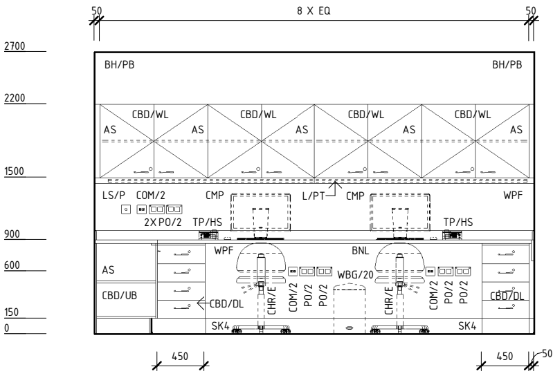
ELEVATION 02
