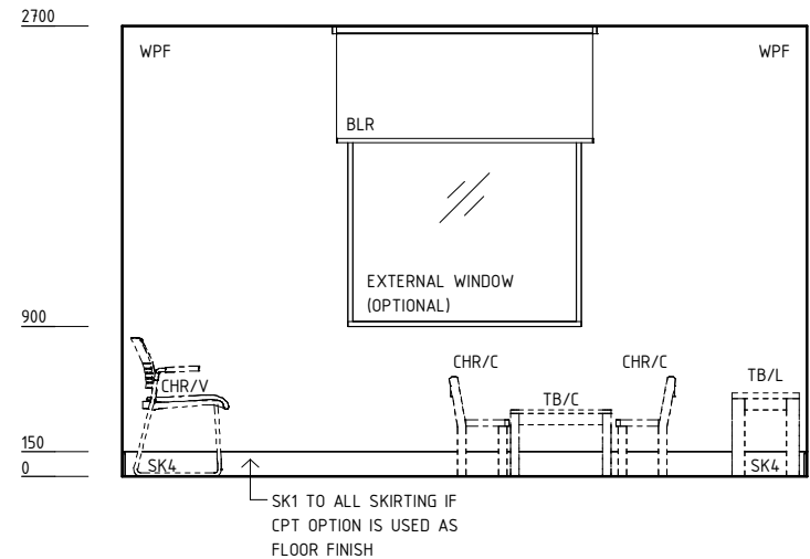
ELEVATION 1
