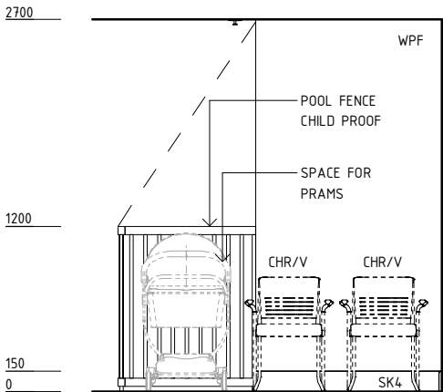
ELEVATION 4
